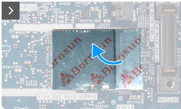
Abbildung 17. Einbauen des 2230-Solid-State-Laufwerks
