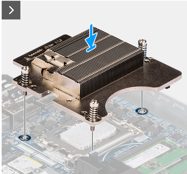
Abbildung 69. Einsetzen des Kühlkörpers
