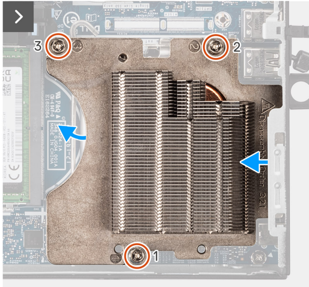
Abbildung 68. Kühlkörper entfernen
