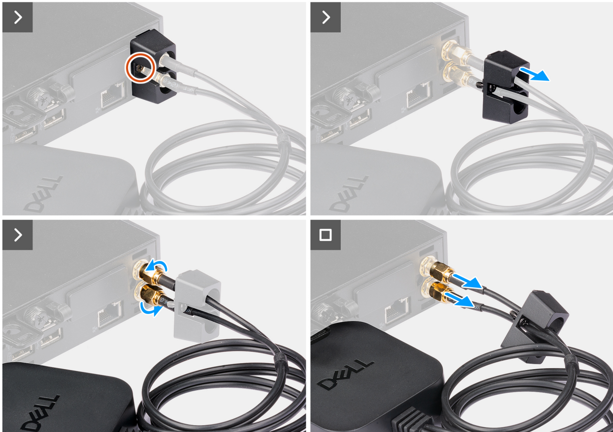
Abbildung 34. Entfernen der externen Puck-Antenne
