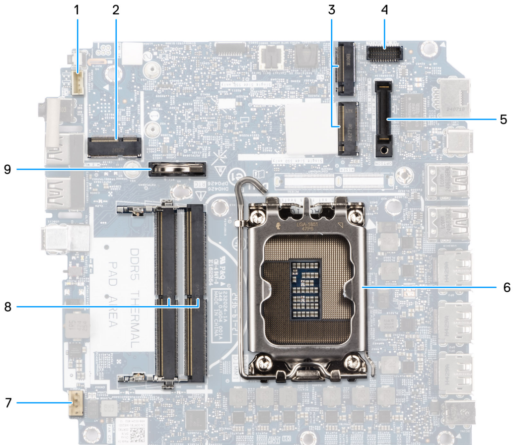
Abbildung 80. Anschlüsse auf der Hauptplatine
