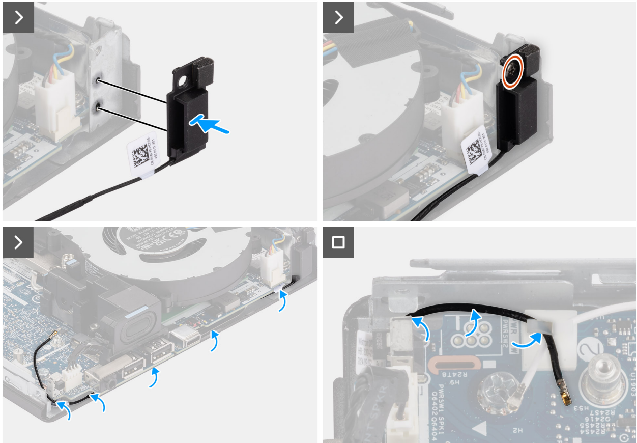
Abbildung 71. Einbauen des Antennenmoduls (schwarzes Kabel)
