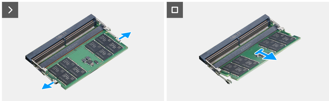
Abbildung 32. Entfernen des Arbeitsspeichermoduls
