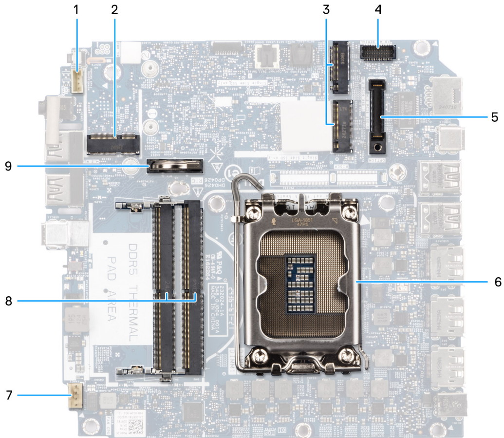
Abbildung 83. Anschlüsse auf der Hauptplatine
