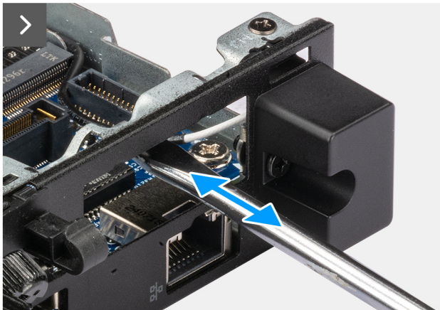
Abbildung 39. Installieren des dualen USB-3.2-Gen2-Anschlussmoduls
