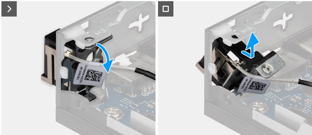
Abbildung 73. Entfernen des Antennenmoduls (weißes Kabel)
