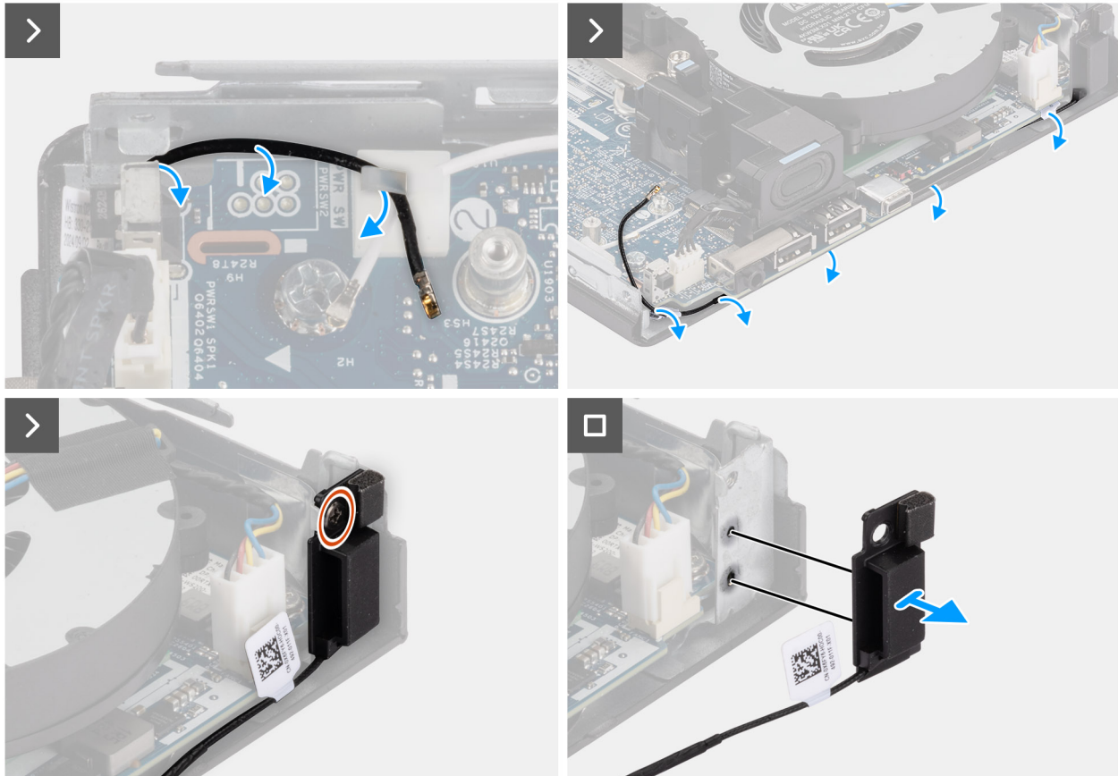
Abbildung 70. Entfernen des Antennenmoduls (schwarzes Kabel)
