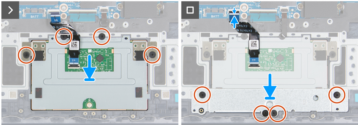
Abbildung 45. Installieren des Touchpads
