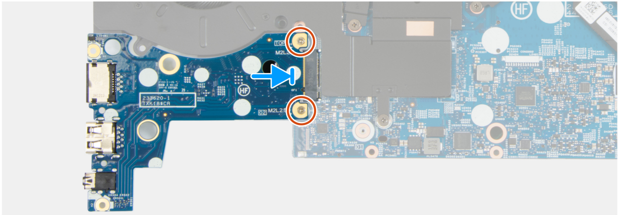
Abbildung 64. Installieren der I/O-Platine
