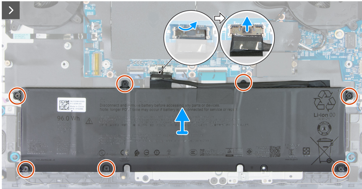
Abbildung 18. Entfernen des Akkus
