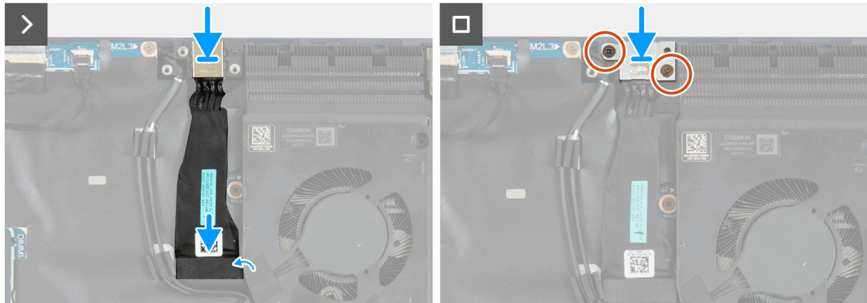
Abbildung 39. Einbauen des Netzadapteranschlusses
