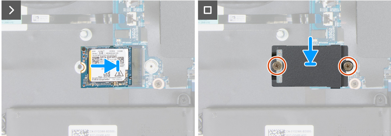
Abbildung 27. Installieren des M.2 2230-SSD im Steckplatz SSD2
