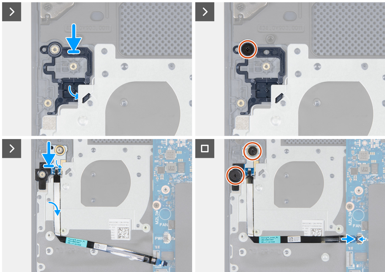
Abbildung 60. Einbauen des Netzschalters und der Netzschalterplatine
