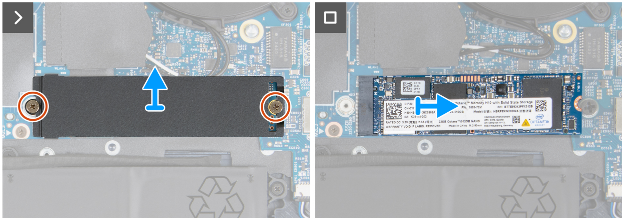
Abbildung 28. Entfernen des M.2 2280-SSD-Laufwerks aus dem Steckplatz SSD1
