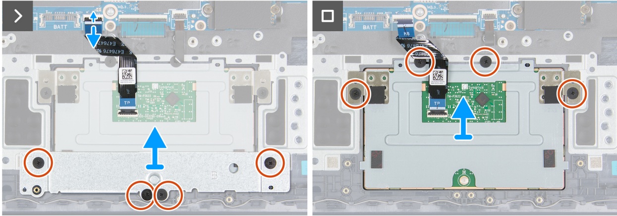
Abbildung 44. Entfernen des Touchpads
