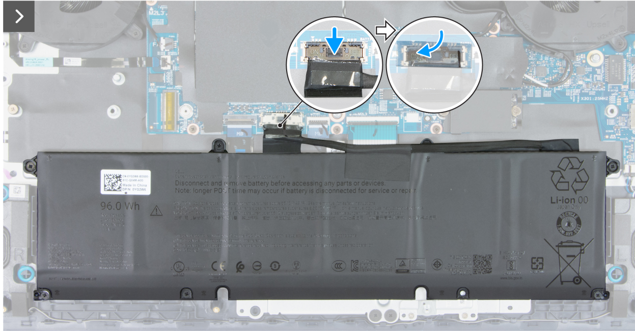
Abbildung 15. Verbinden des Akkukabels
