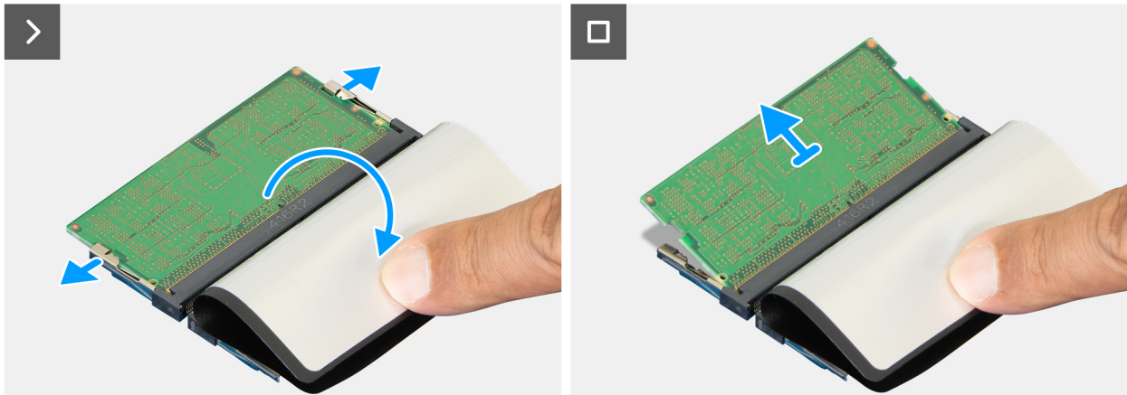
Abbildung 22. Entfernen des Arbeitsspeichermoduls
