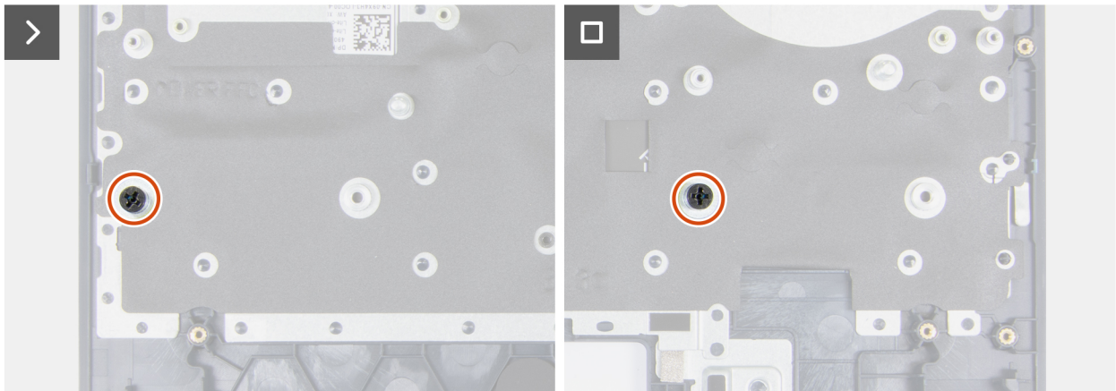
Abbildung 78. SSD-Schraubenhalterungen entfernen
