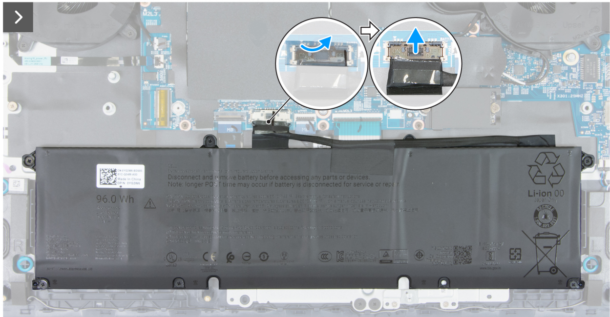
Abbildung 14. Trennen des Akkukabels
