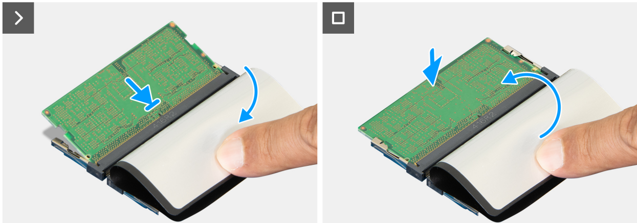
Abbildung 23. Einsetzen des Speichermoduls
