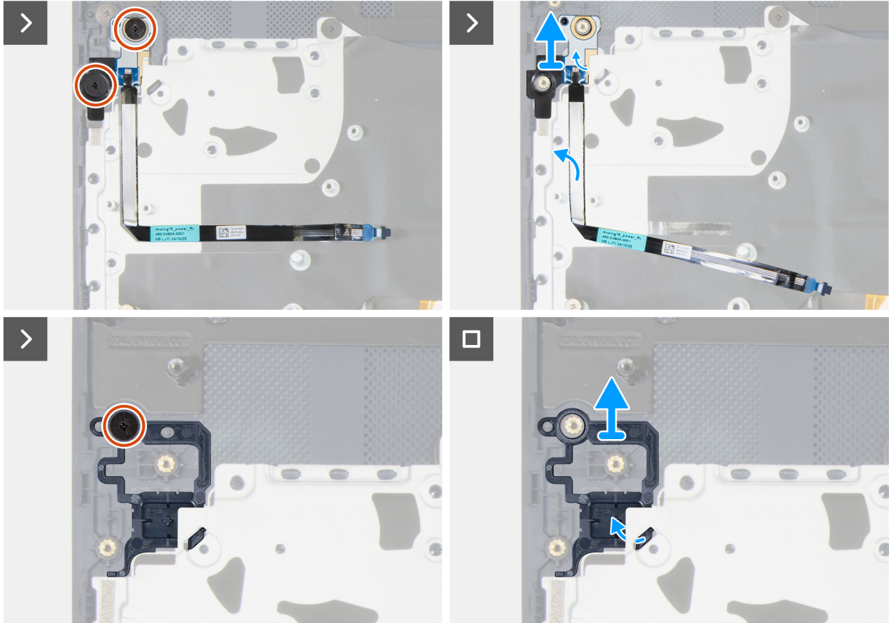
Abbildung 58. Entfernen des Netzschalters und der Netzschalterplatine
