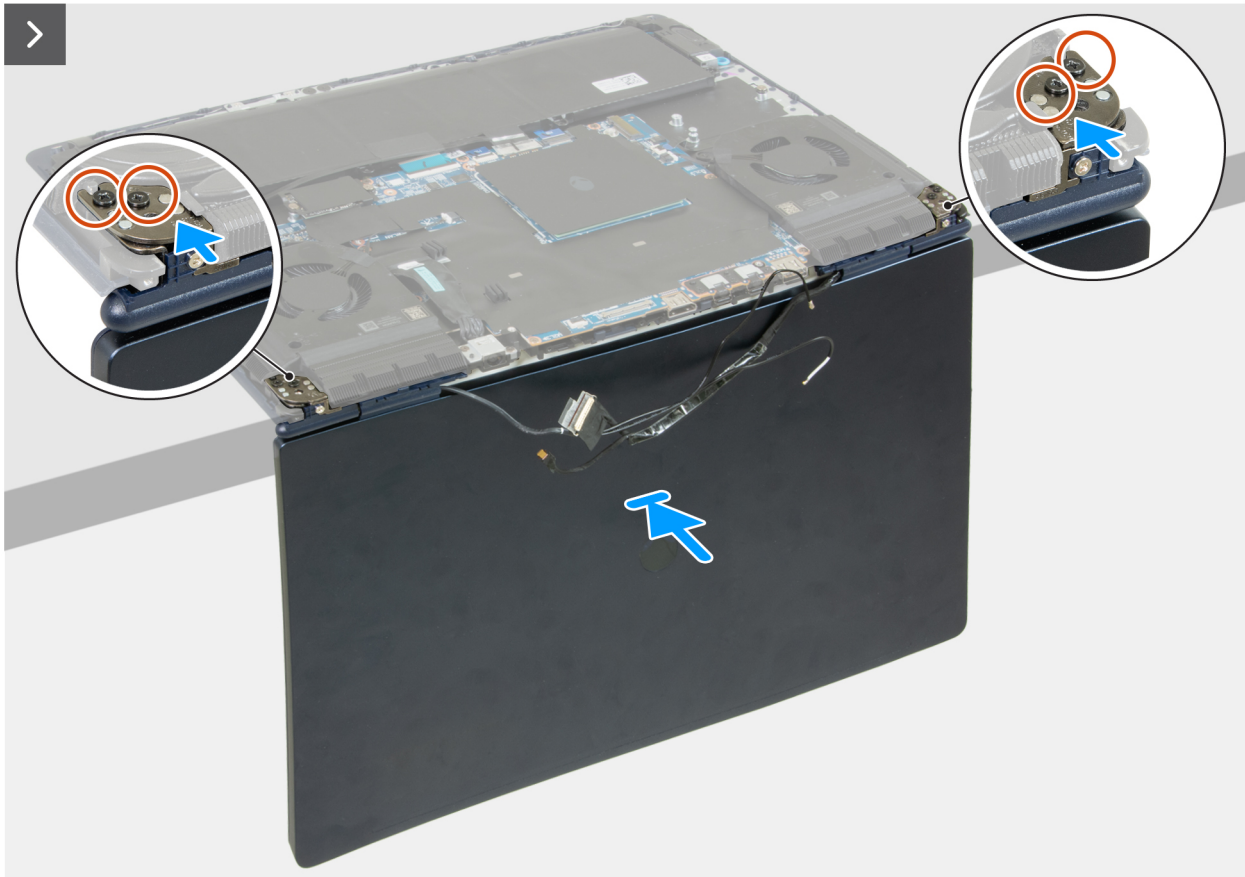
Abbildung 75. Einbauen der Bildschirmbaugruppe
