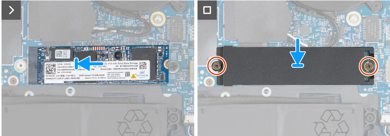
Abbildung 29. Installieren des M.2 2280-SSD-Laufwerks im Steckplatz SSD1
