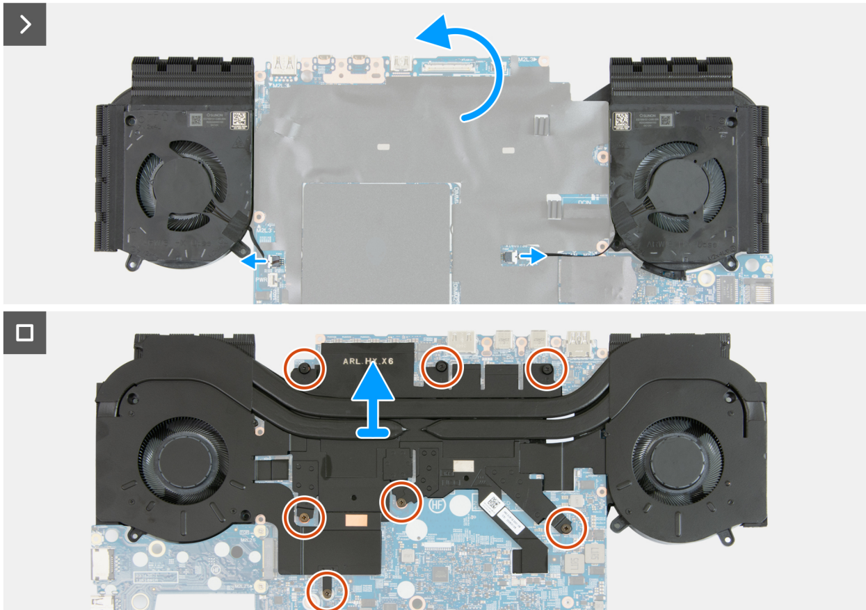
Abbildung 51. Entfernen der Hauptplattenbaugruppe.
