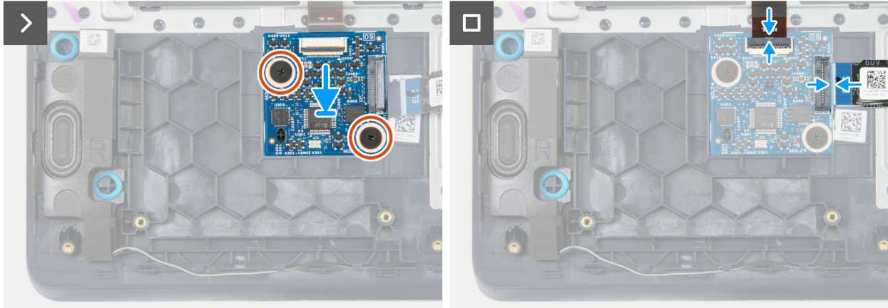
Abbildung 47. Einbauen der Platine des Controllers für die Tastaturhintergrundbeleuchtung (ELC)
