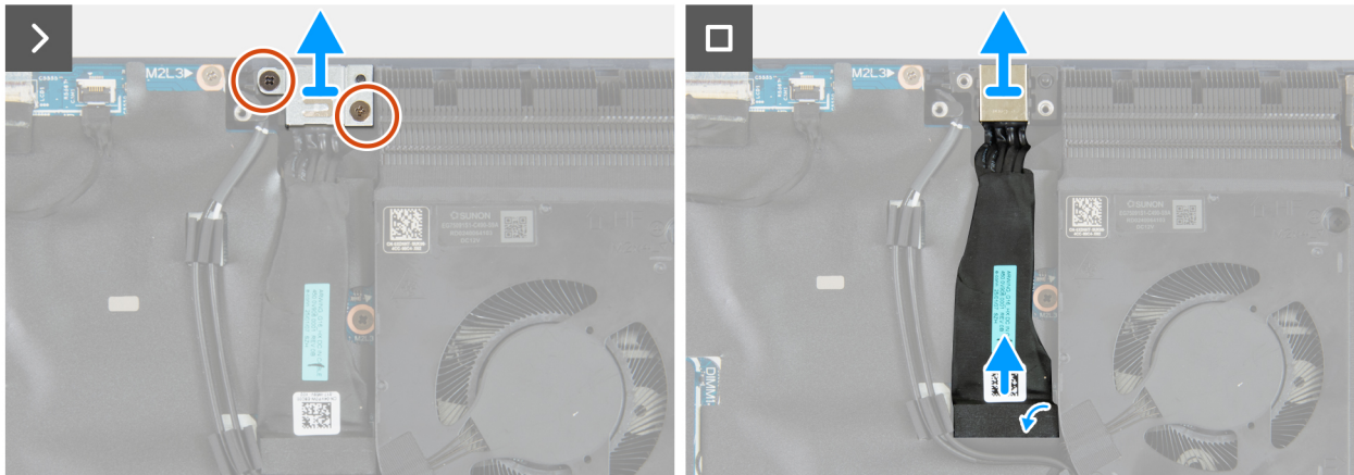
Abbildung 38. Entfernen des Netzadapteranschlusses
