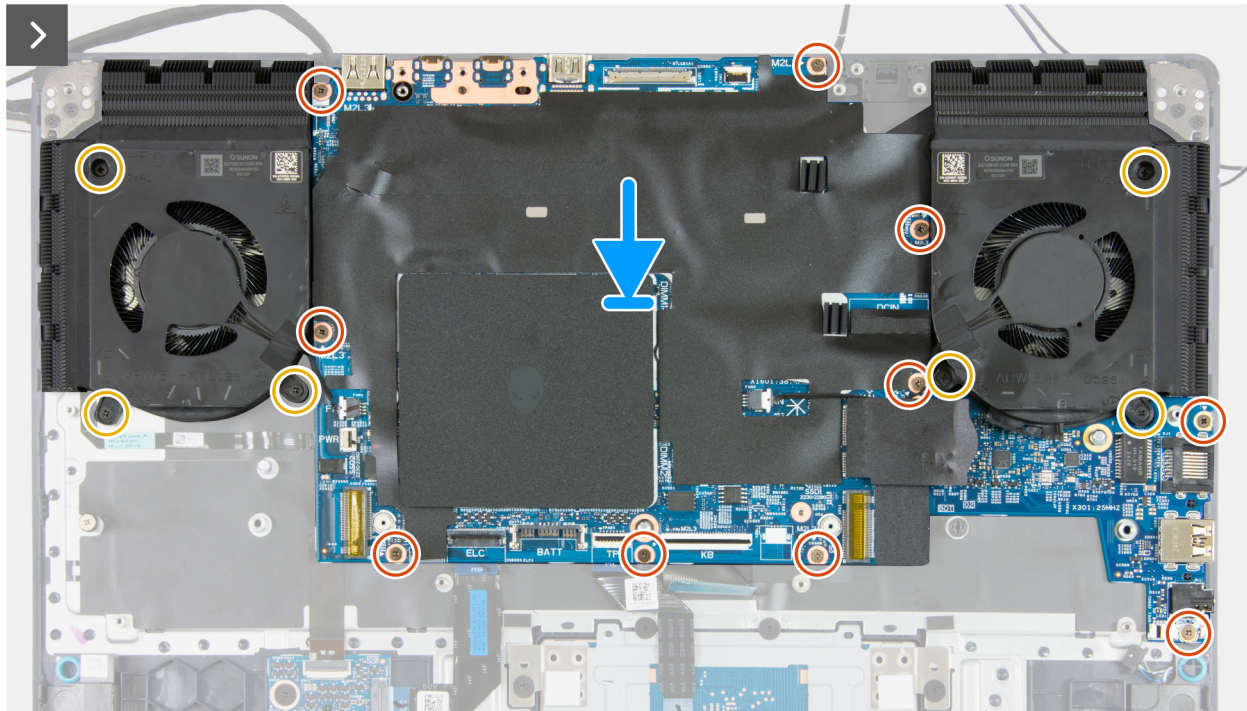
Abbildung 56. Einbauen der Systemplatine
