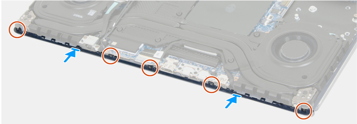
Abbildung 67. Anbringen der rückseitigen Abdeckung
