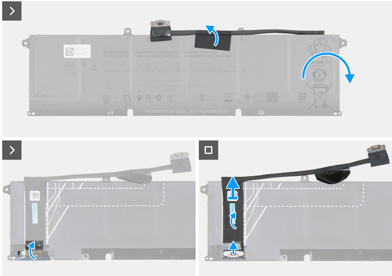
Abbildung 20. Entfernen des Kabels des Akkus
