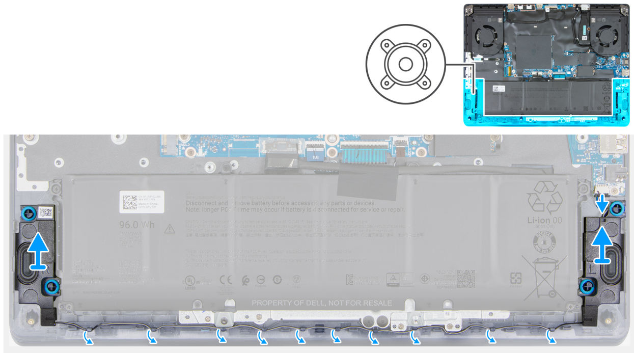
Abbildung 36. Entfernen der Lautsprecher
