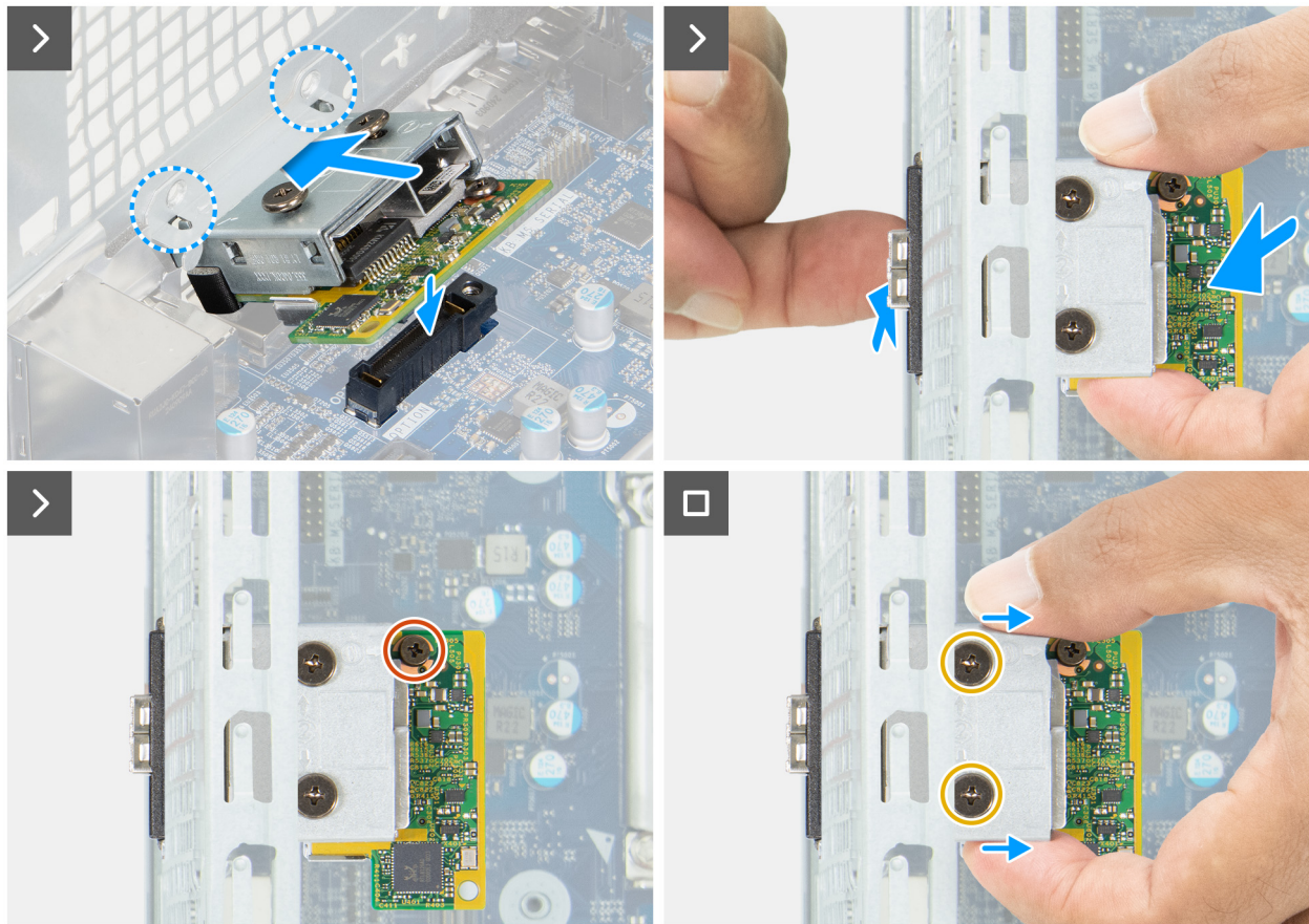
Abbildung 80. Installieren des Fiberoptik-Port-Moduls
