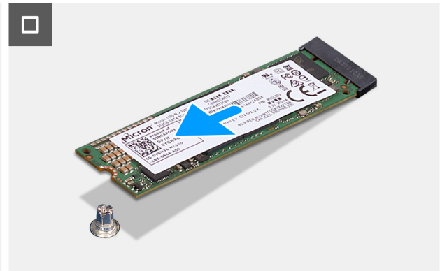
Abbildung 31. Entfernen des M.2 2280-Solid-State-Laufwerks aus Steckplatz 0
